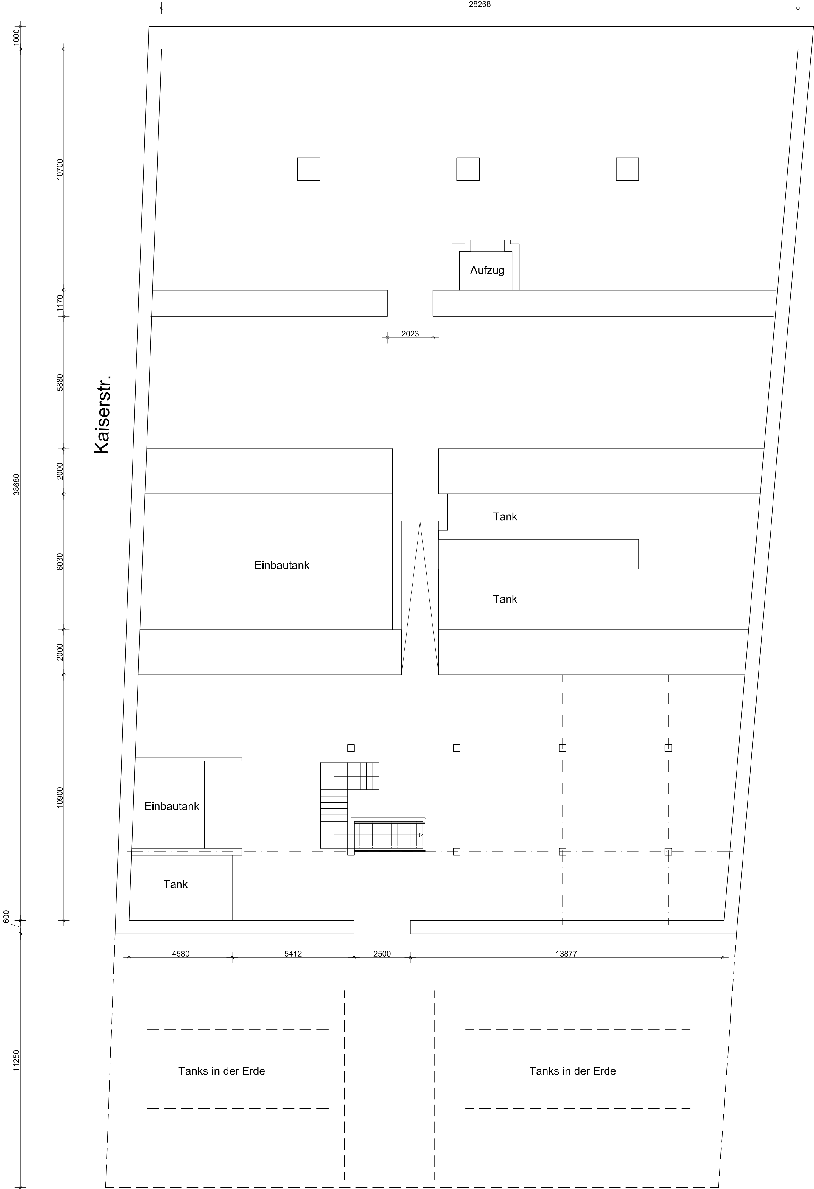
2. Untergeschoss 1:100
