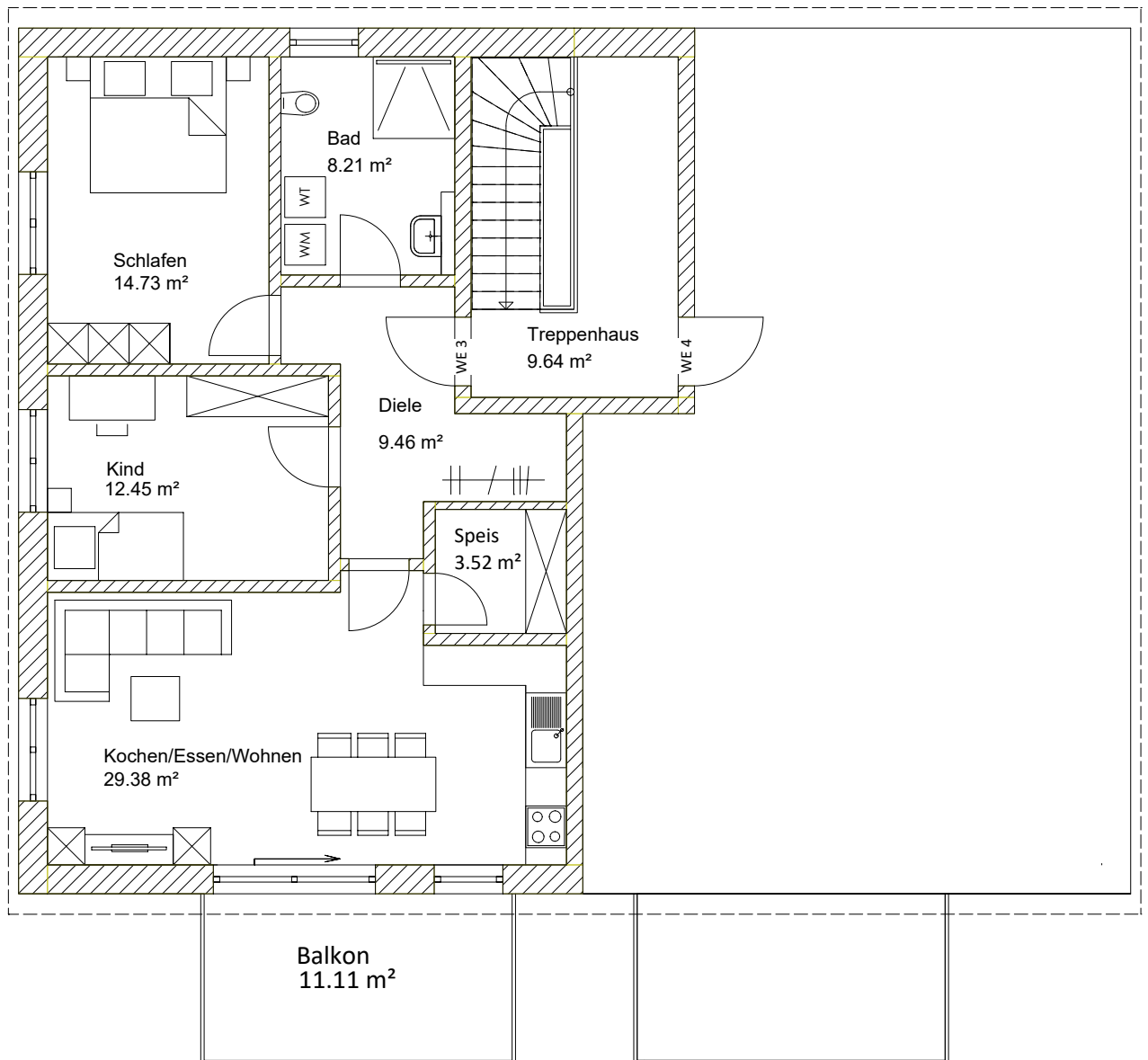
Obergeschoss Wohneinheit 3
