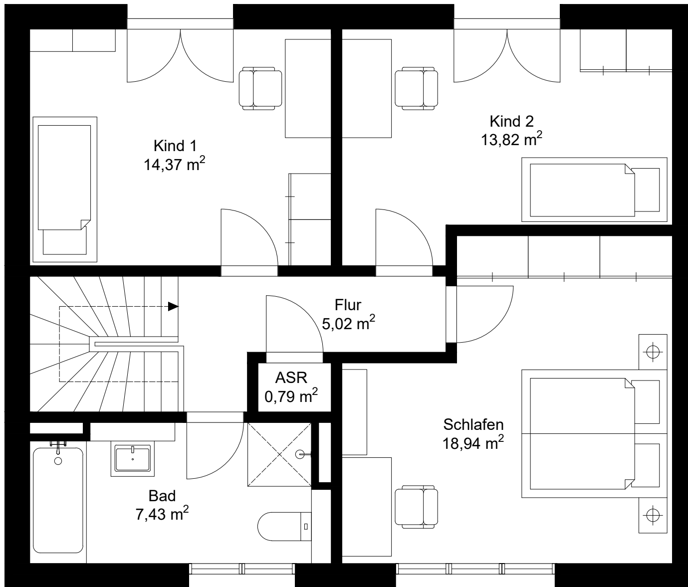
Grundriss Obergeschoss
