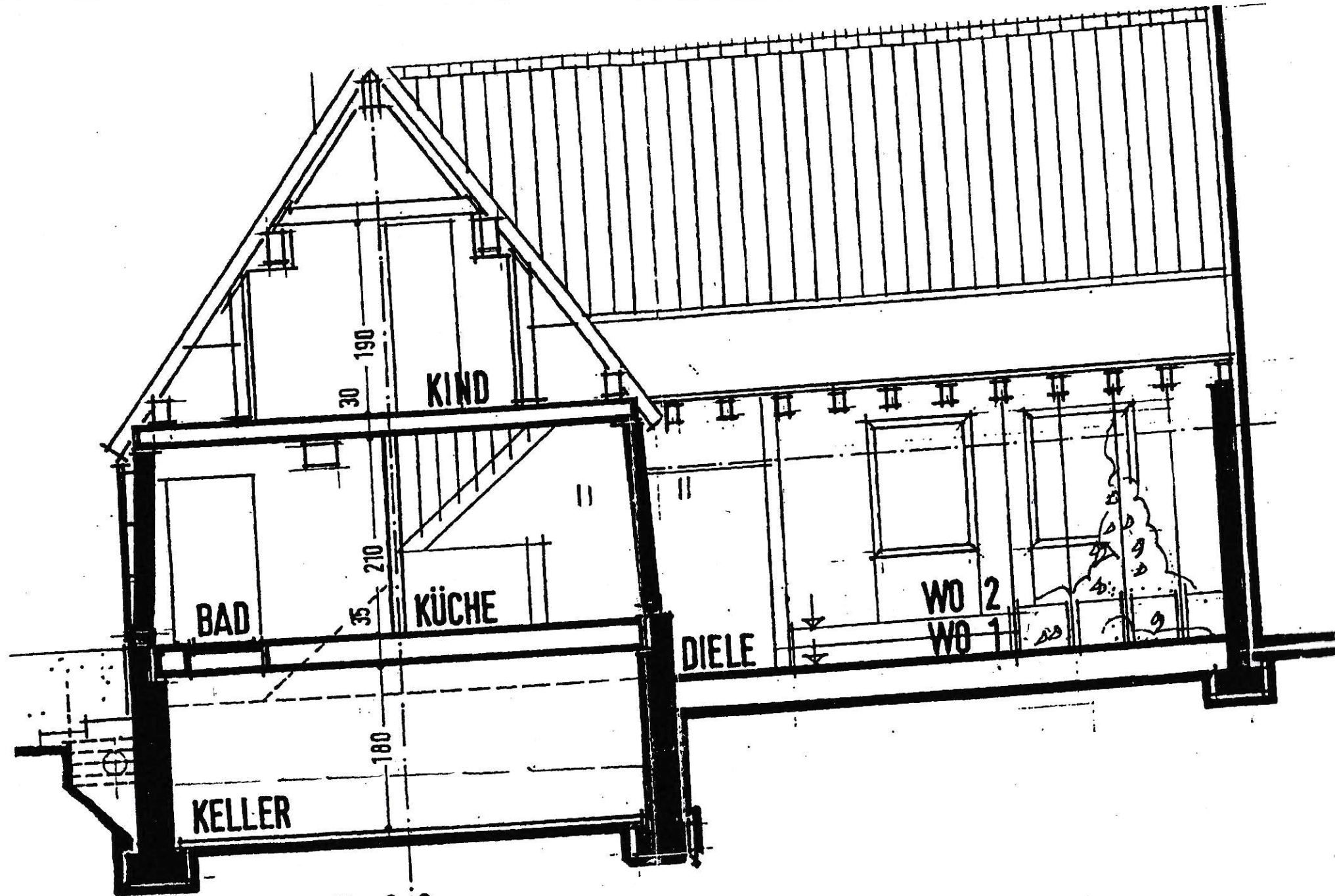
SCHNITT 1:1
