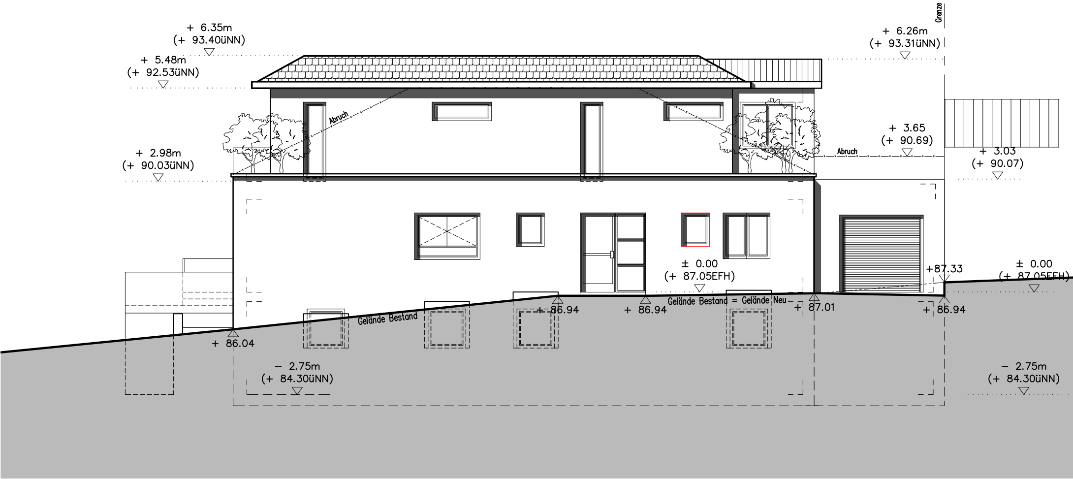
Straßenansicht
