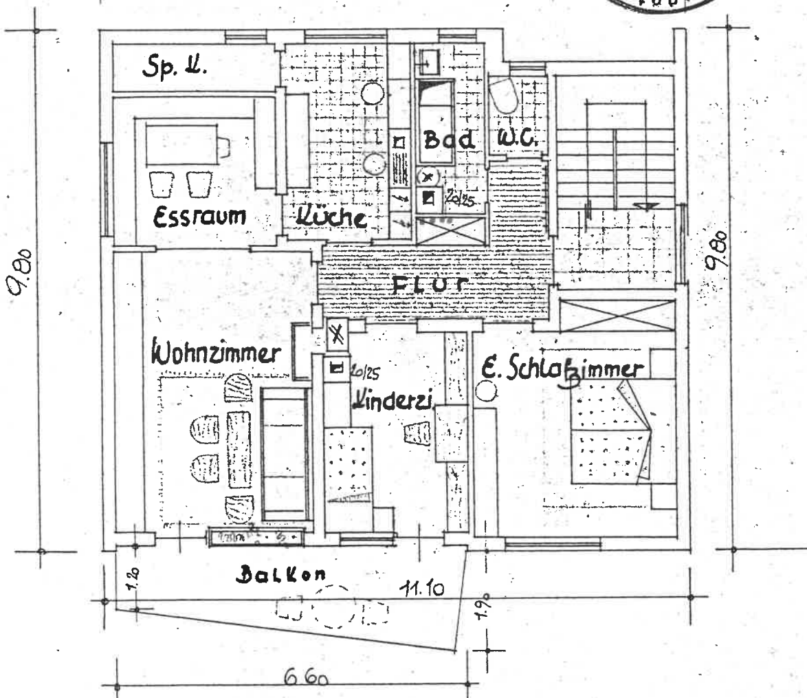
Grundriss I. Stock 1:100 11.10
