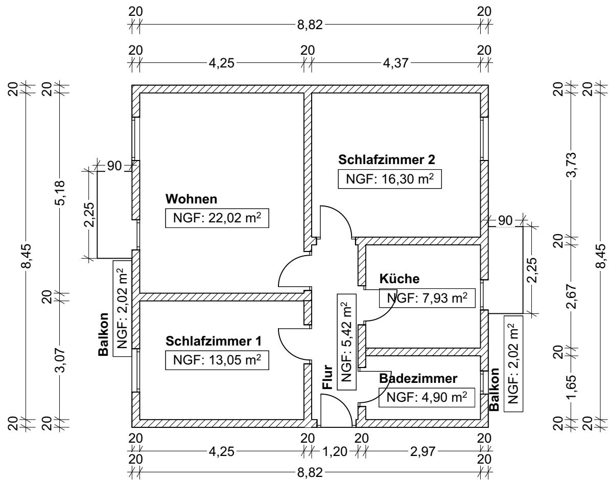
0. Wohnungsgrundriss 1:100
