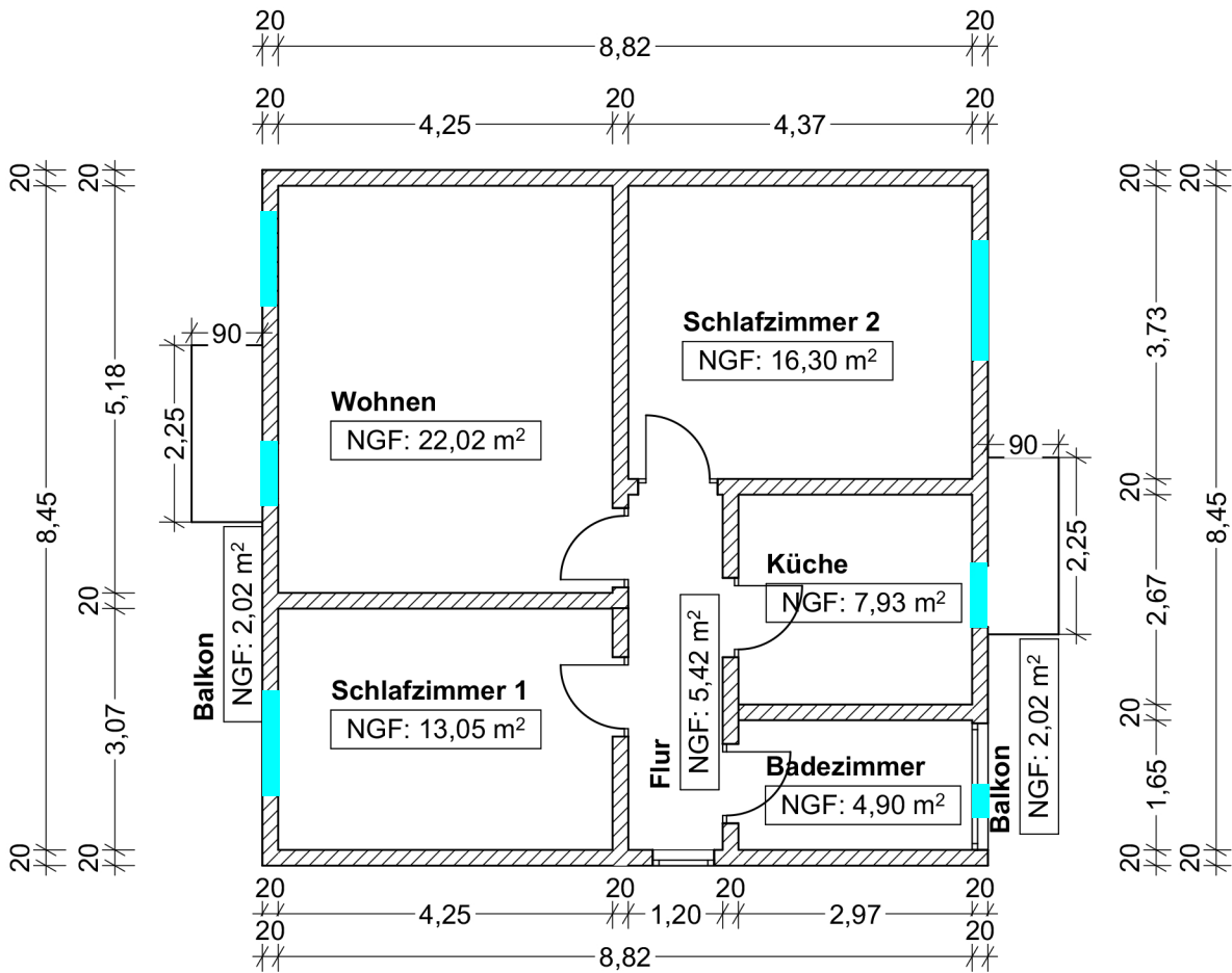
0. Wohnungsgrundriss 1:100
