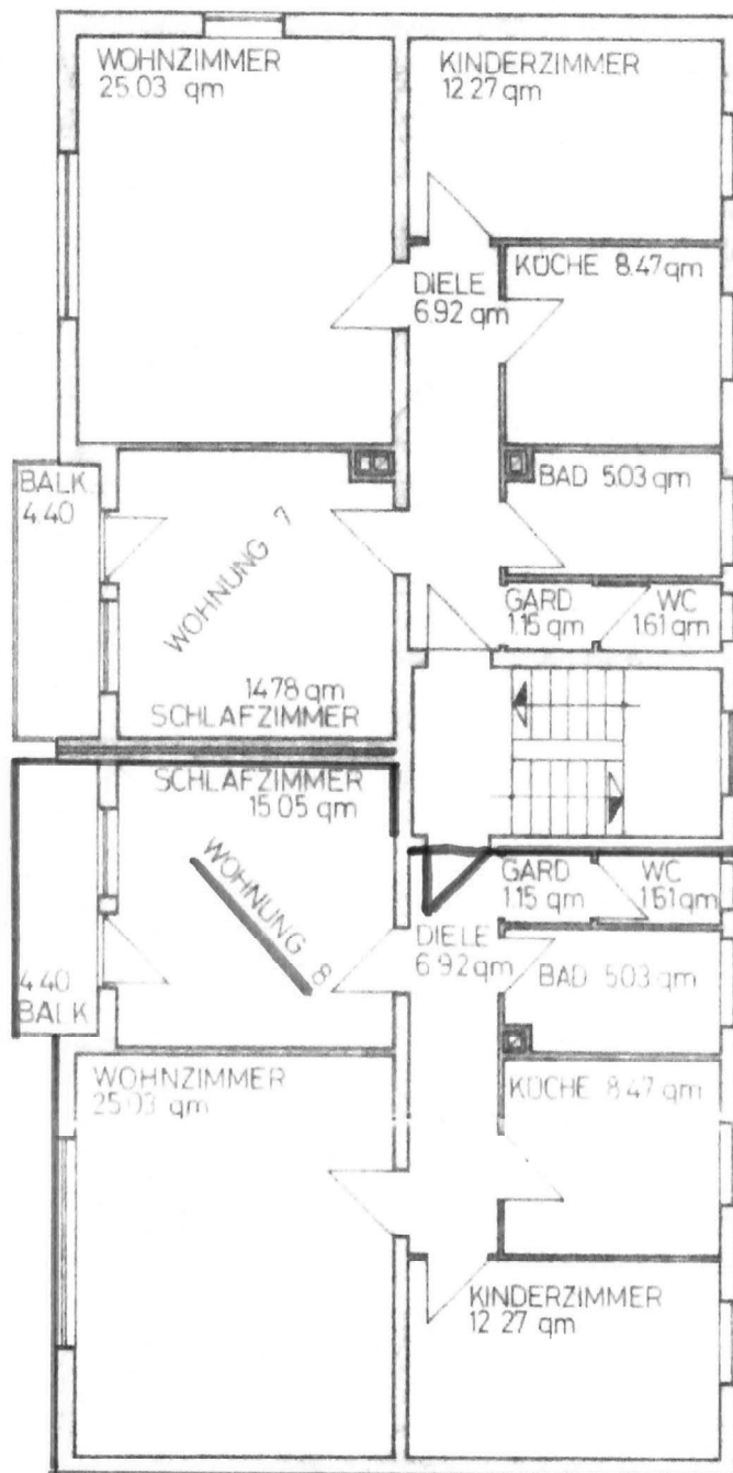
3. OBERGESCHOSS
