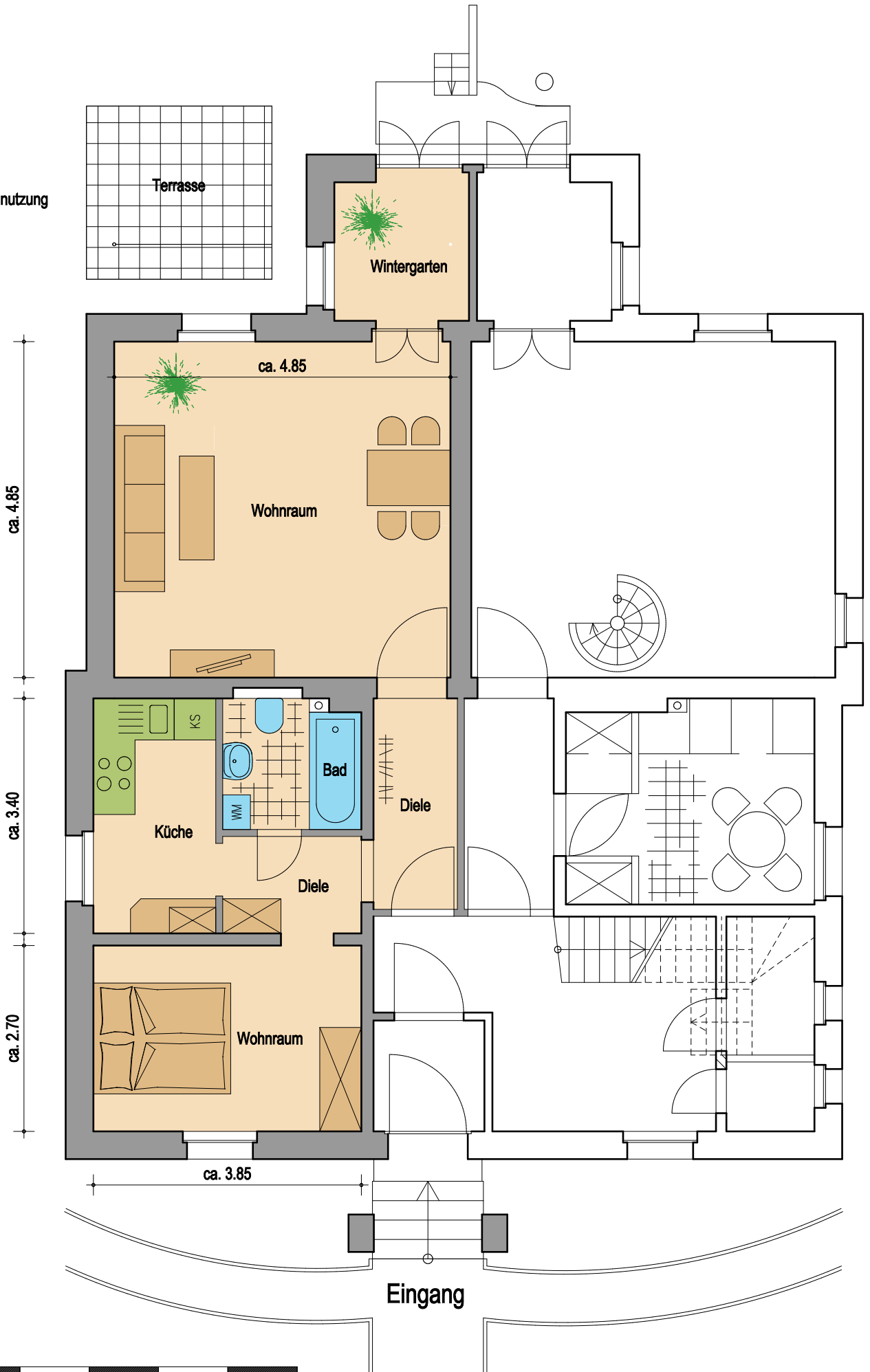
Burgwall 3 - EG - Grundriss Wohnung 1 - 2-Raum - ca. 60.00 m 2 - Maßst.: 1:75
