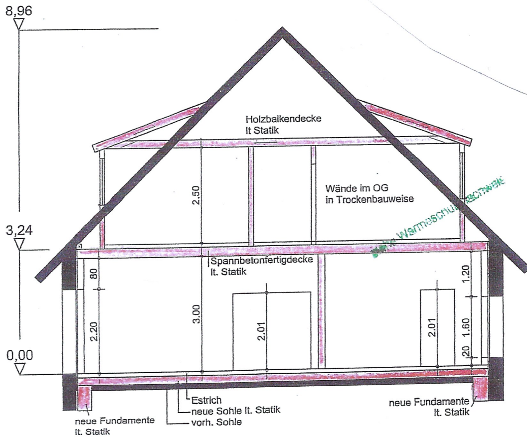
Schnitt A-A
