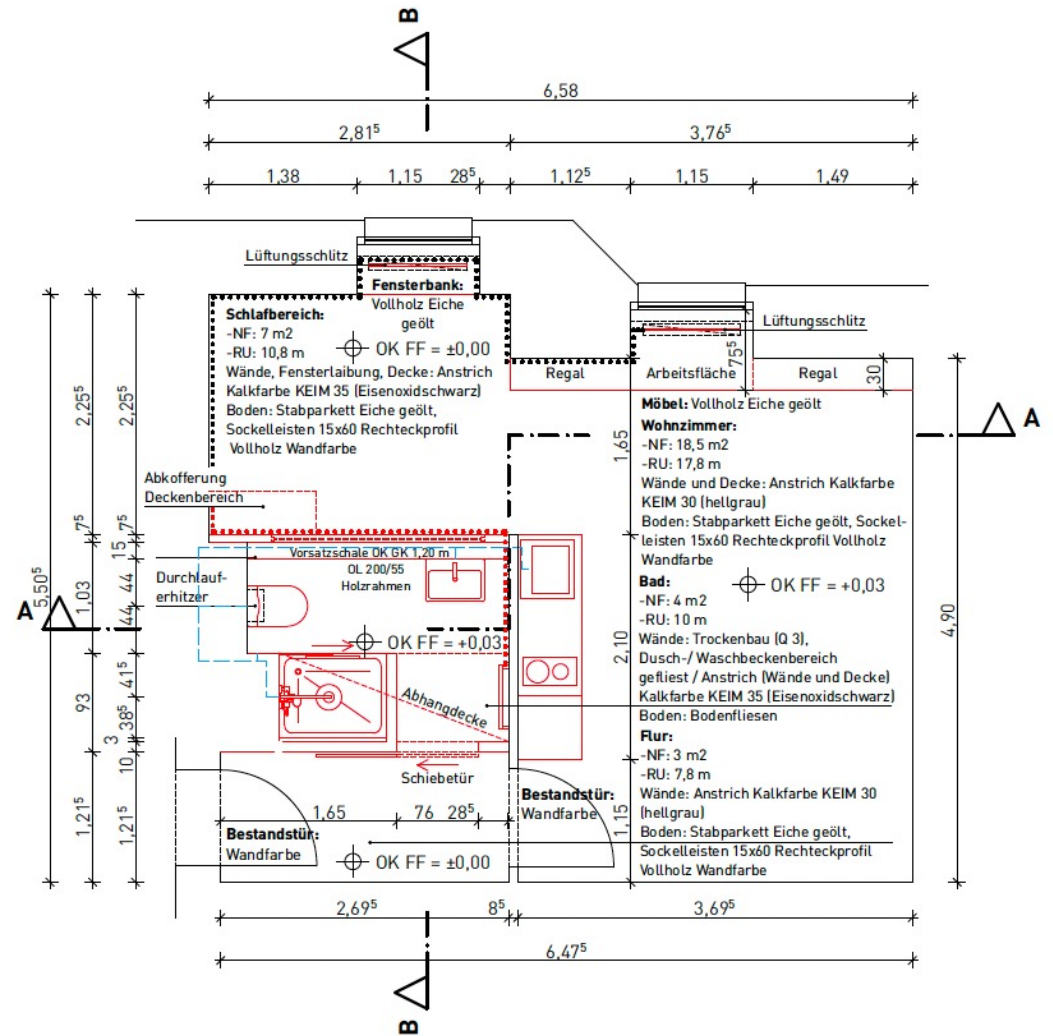
Grundriss Neuplanung
