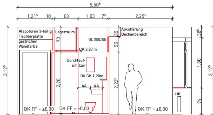
Schnitt B
