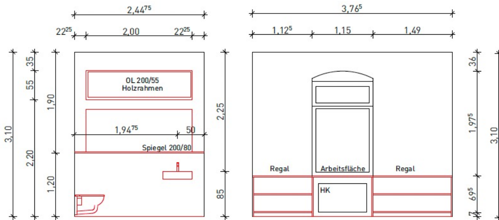
Schnitt A
