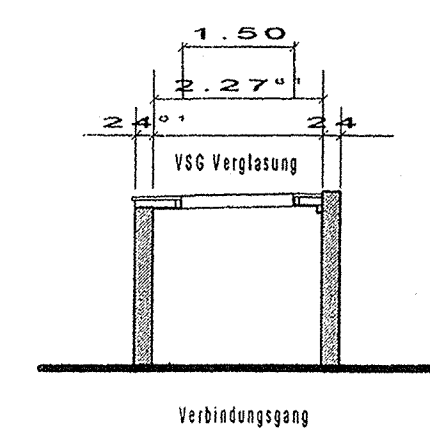
Schnitt A-A 1:100
