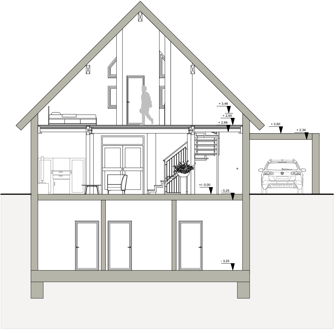
Schnitt A-A
