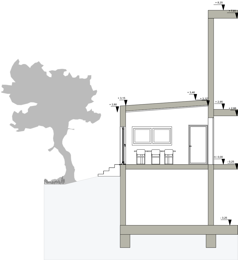
Schnitt B-B
