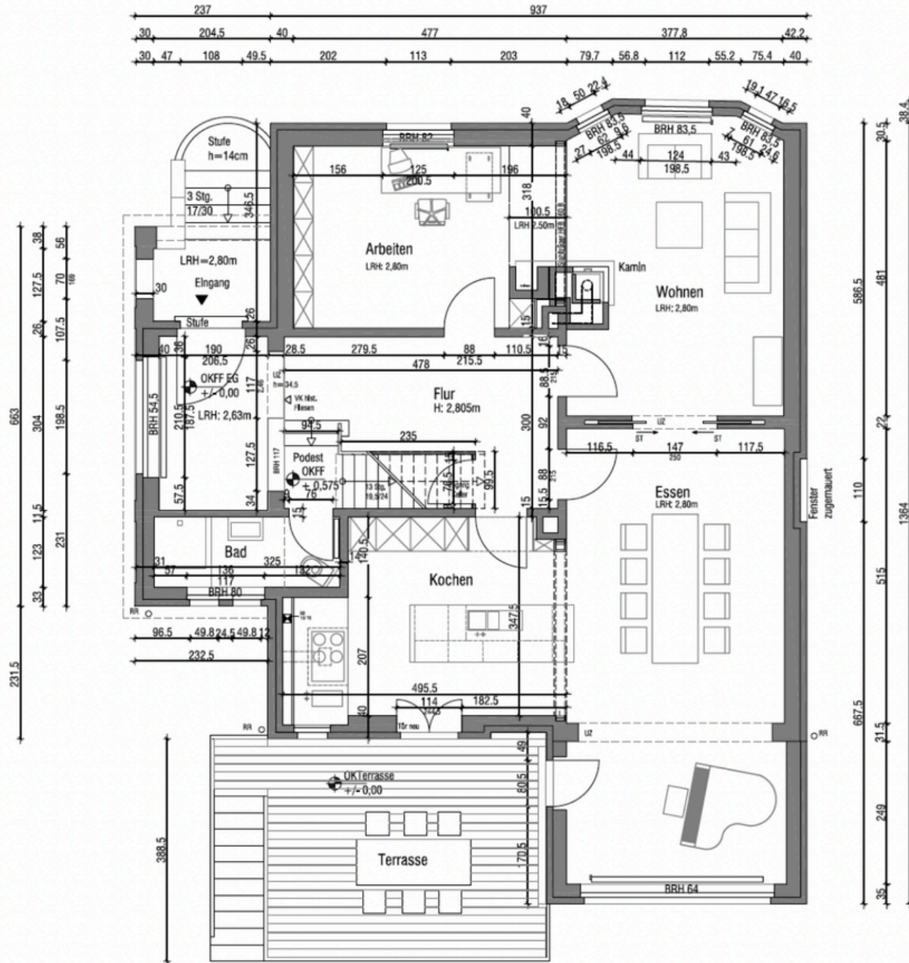
Grundriss Erdgeschoss
