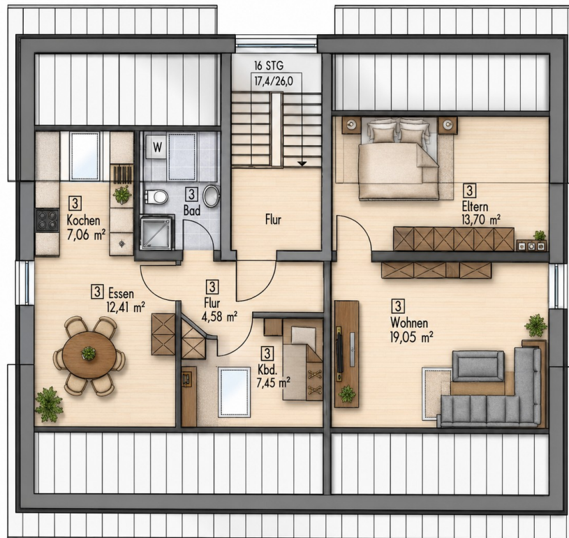
Grundriss
