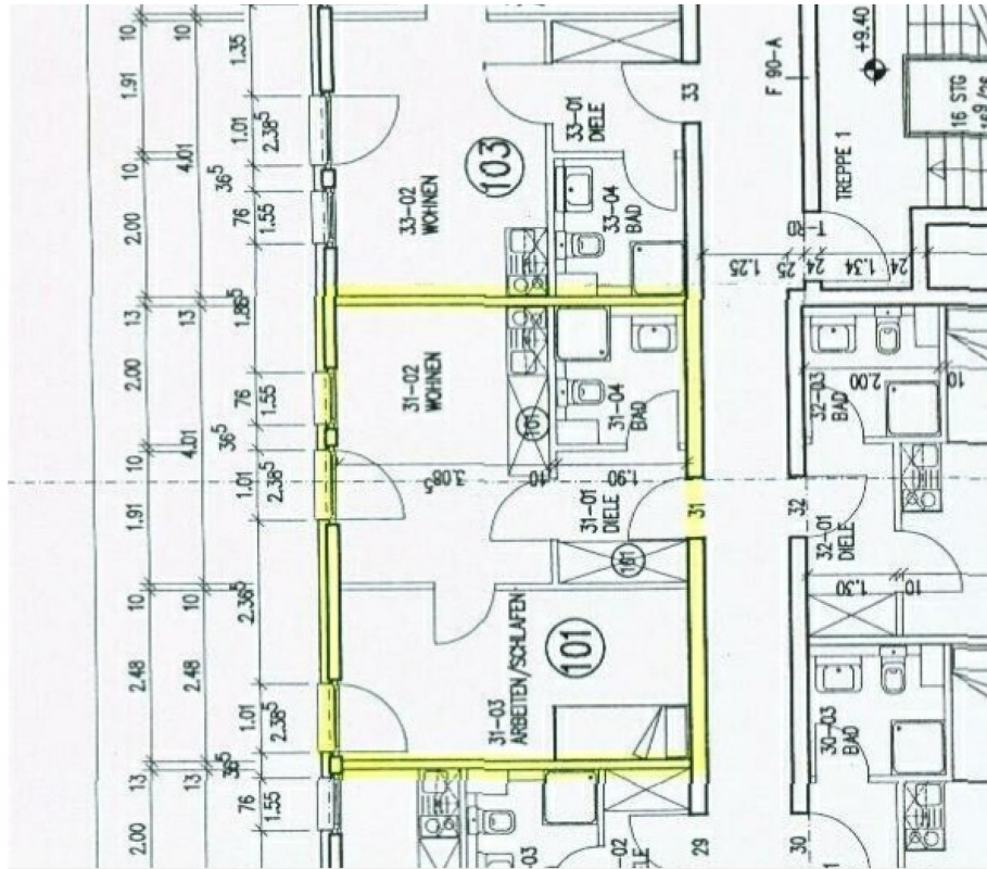
Grundrisse
