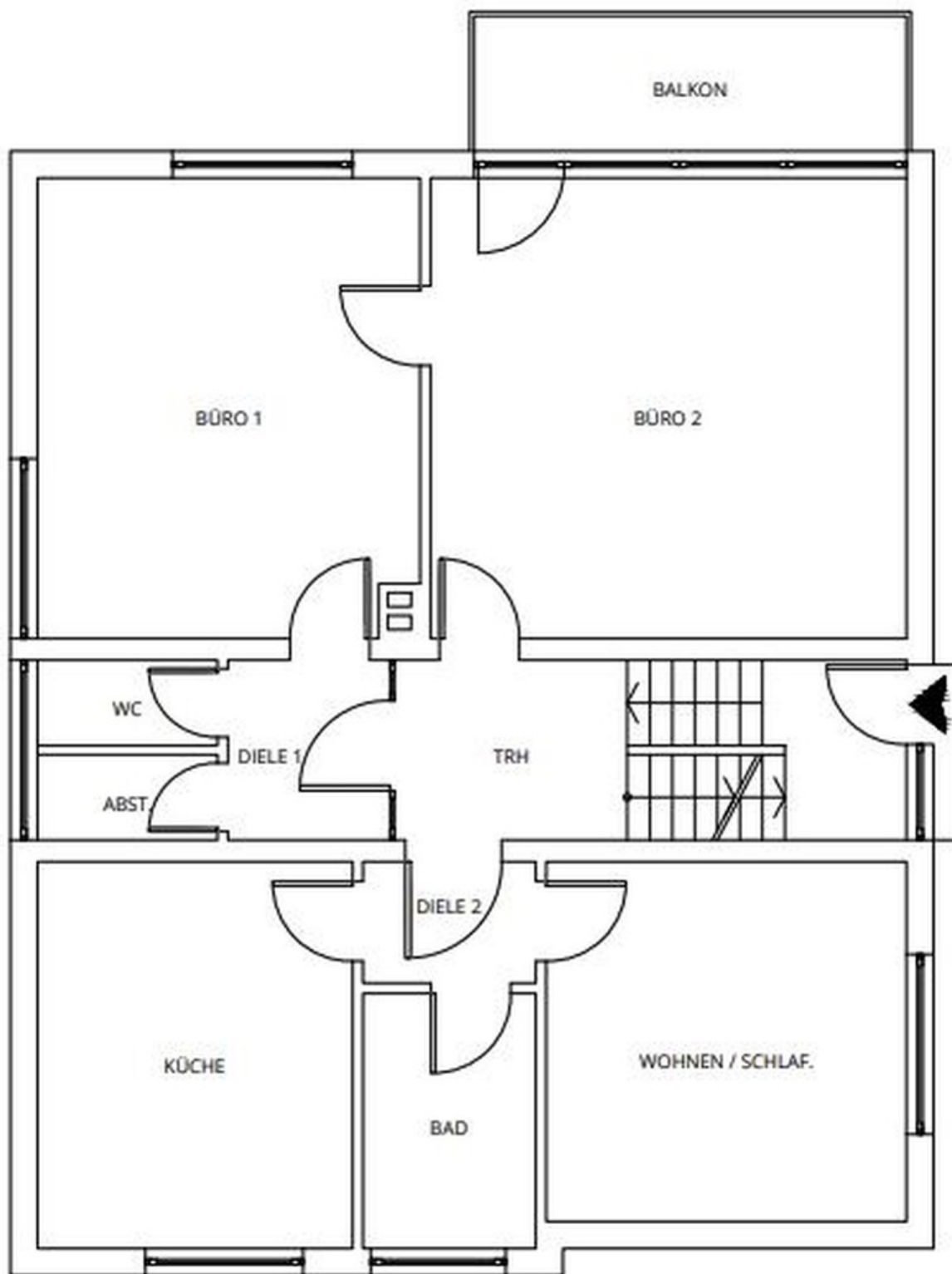
Erdgeschoss
