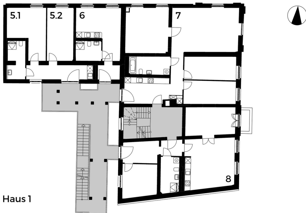
Grundriss Wohnung 08
