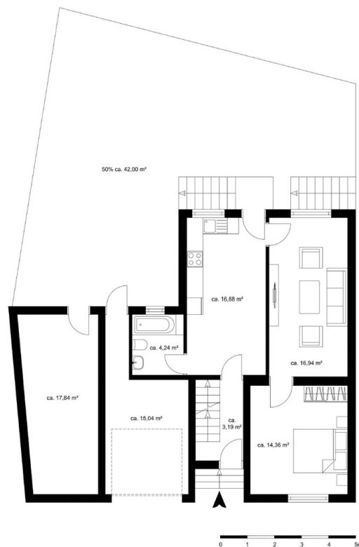
Erdgeschoss
