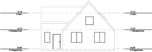
Ostansicht 1:100
