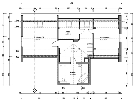
Obergeschoss 1:100
