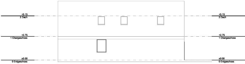
Nordansicht 1:100
