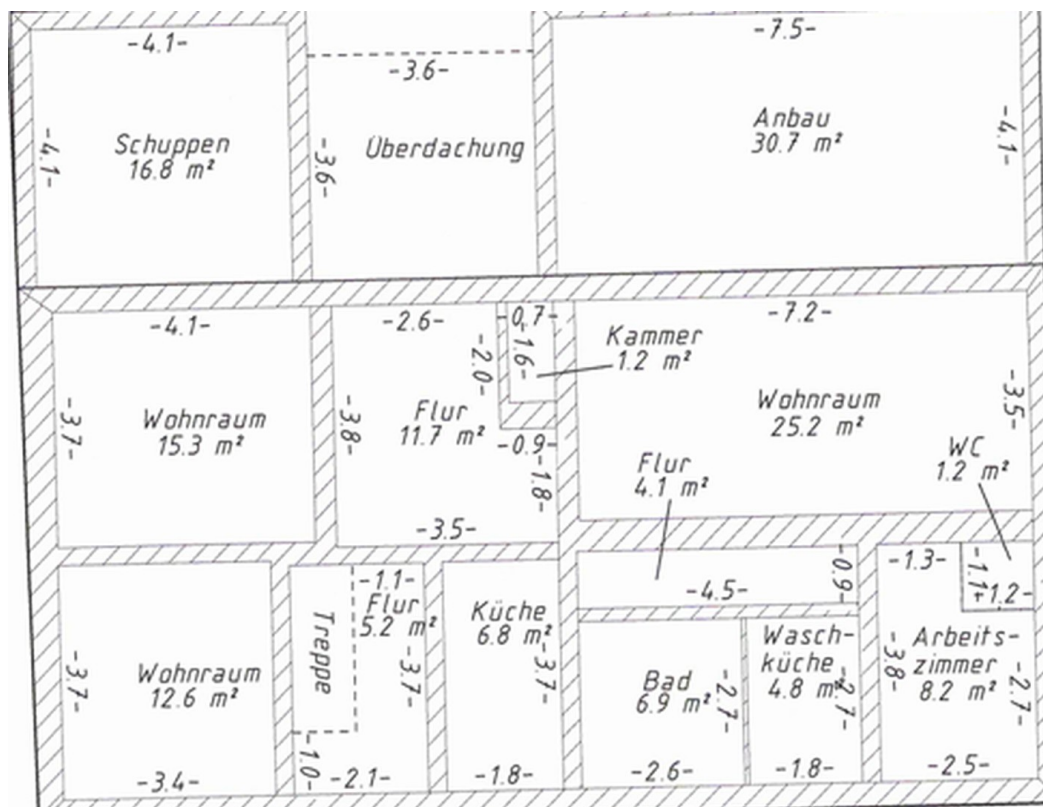
Grundriss Erdgeschoss
