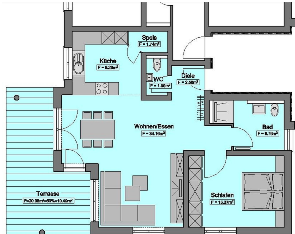
Grundriss
