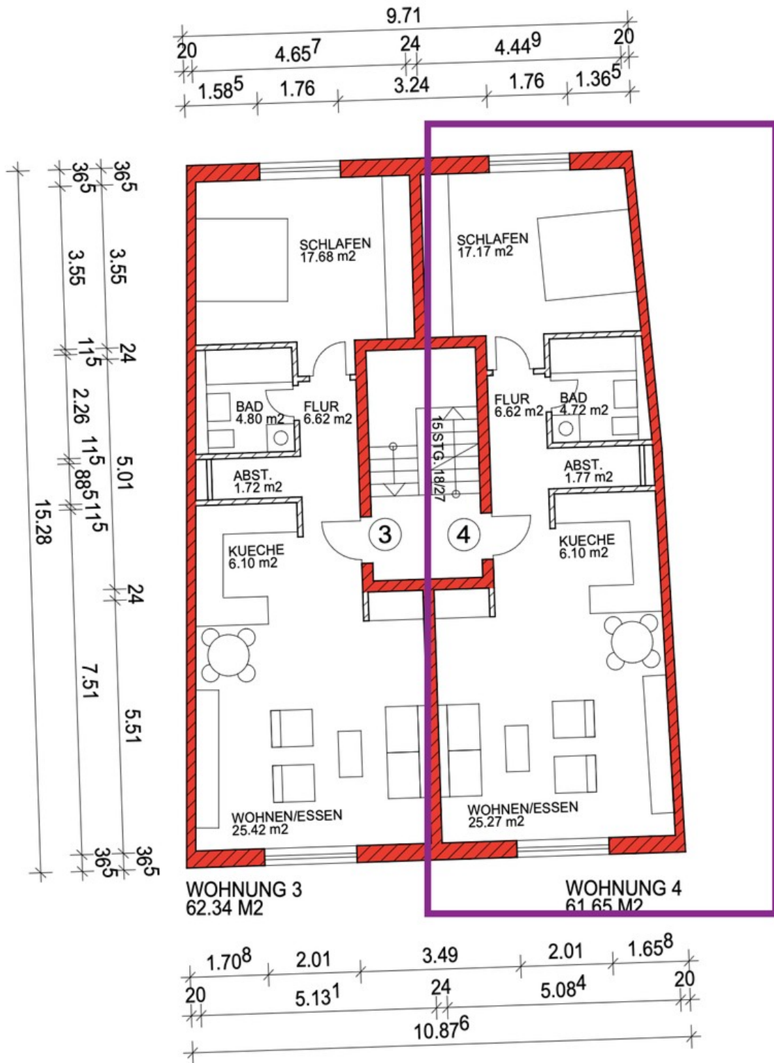
Grundriss
