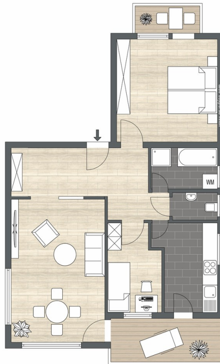
Grundriss
