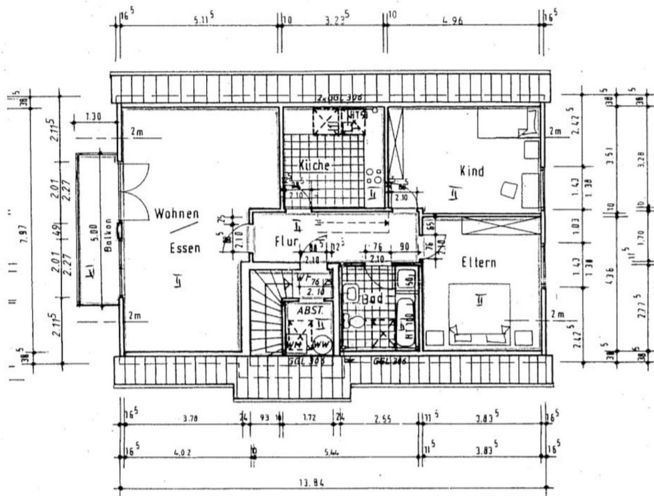
Grundriss
