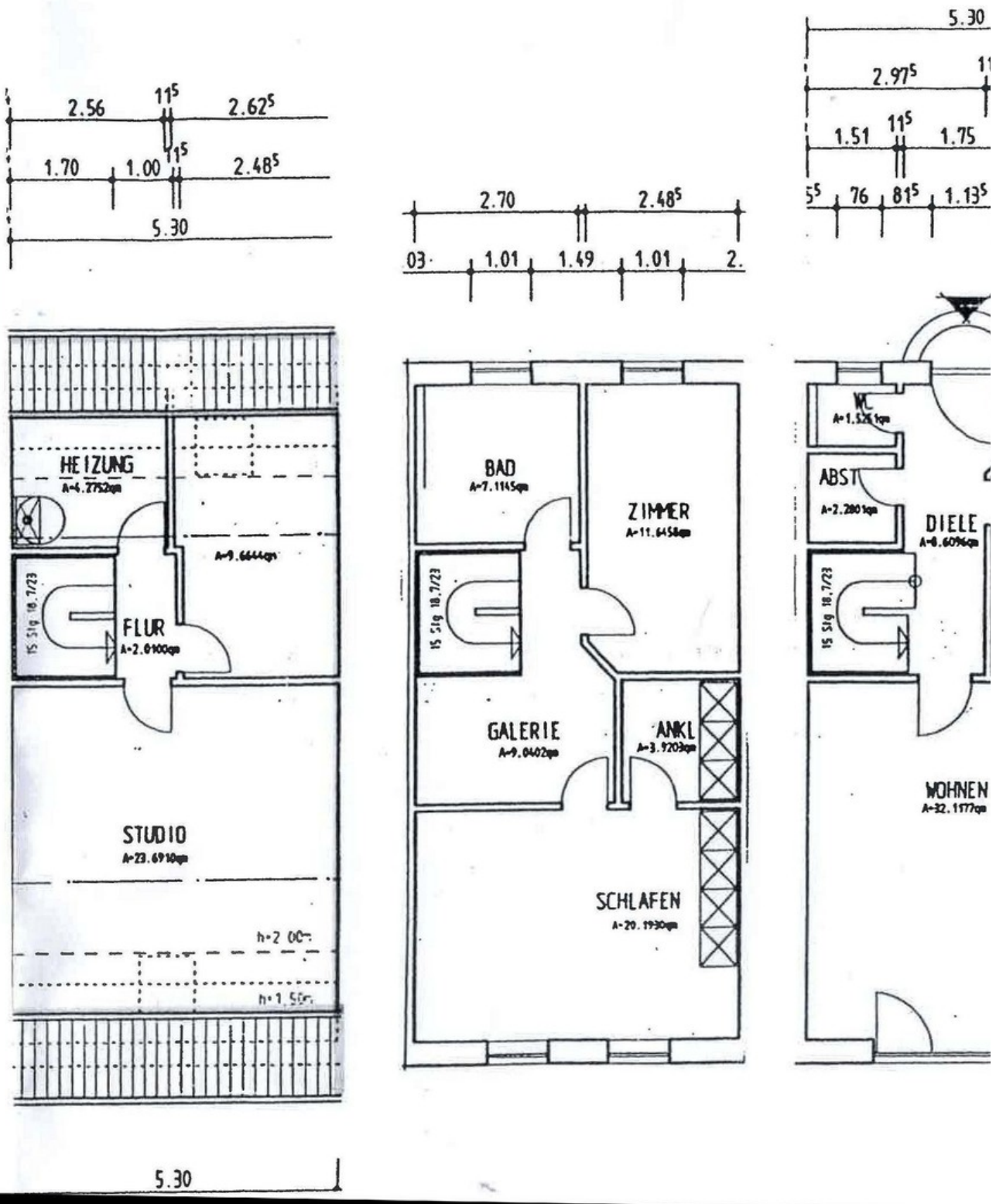
Grundriss
