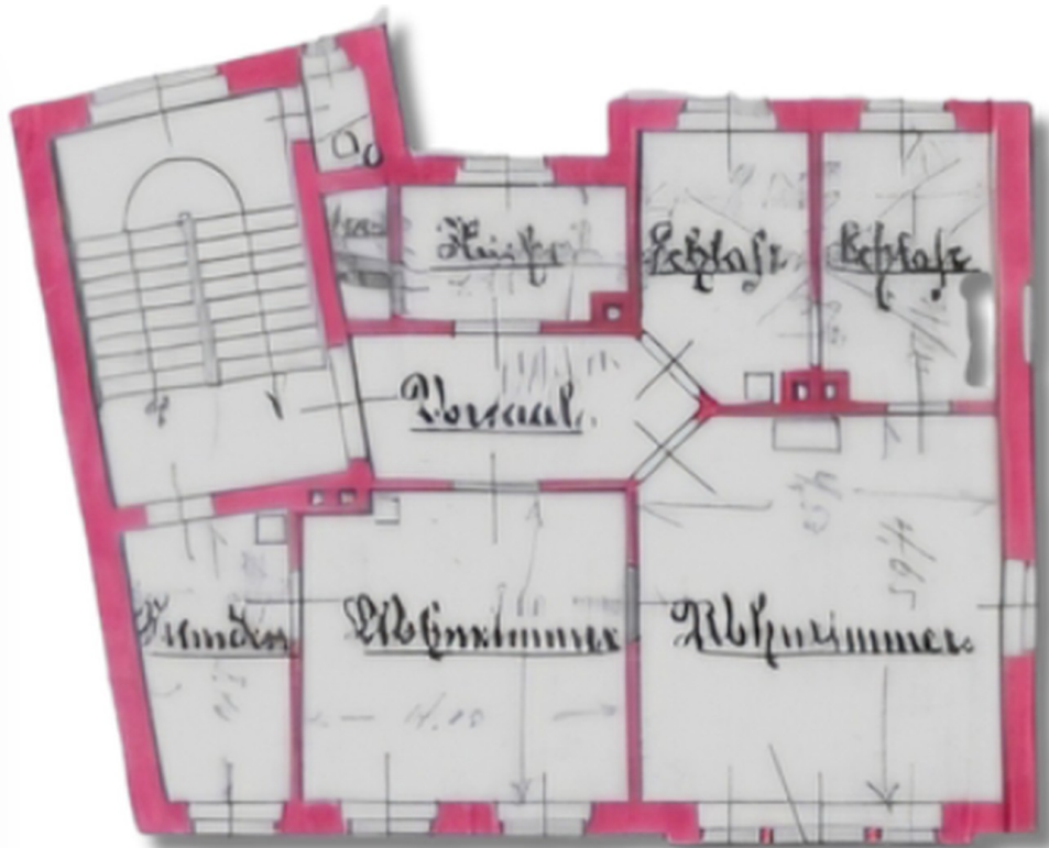
Erdgeschoß (Planung 1890)
