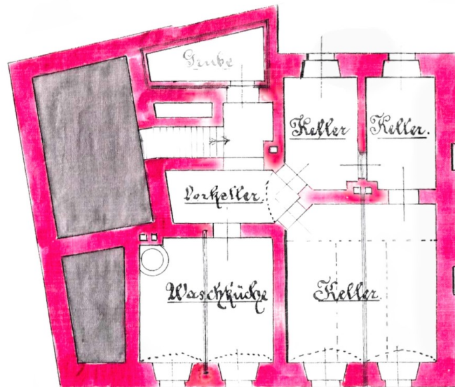
Keller (Planung 1890)
