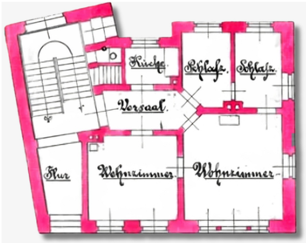
Dachgeschoß (Planung 1890)
