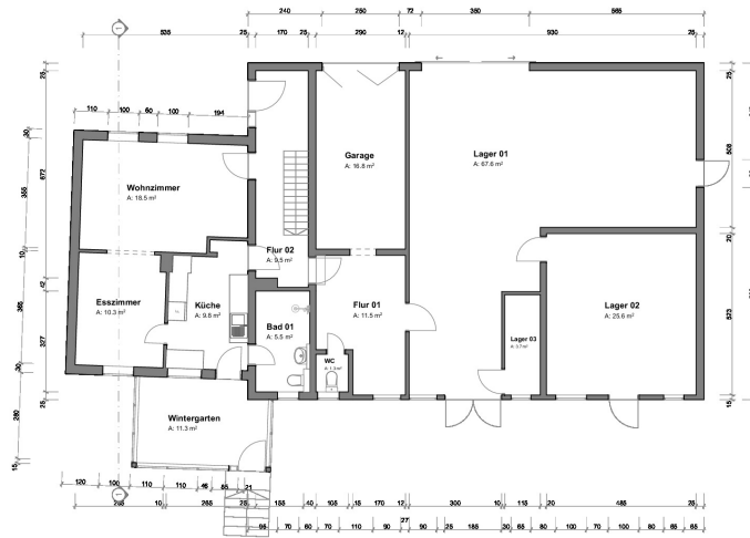
Erdgeschoss 1:100
