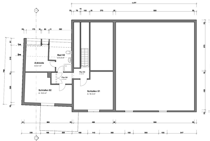
Obergeschoss 1:100
