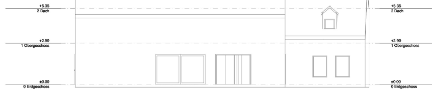
Nordansicht 1:100
