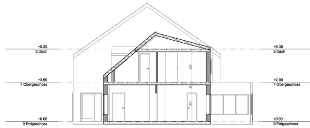
Schnitt 01 1:100
