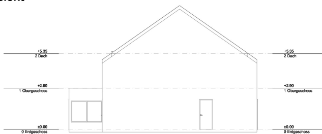
Ostansicht 1:100
