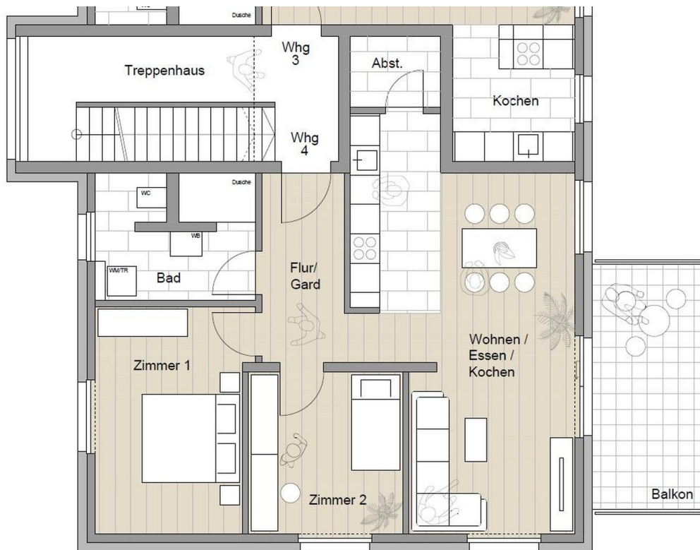
Grundriss
