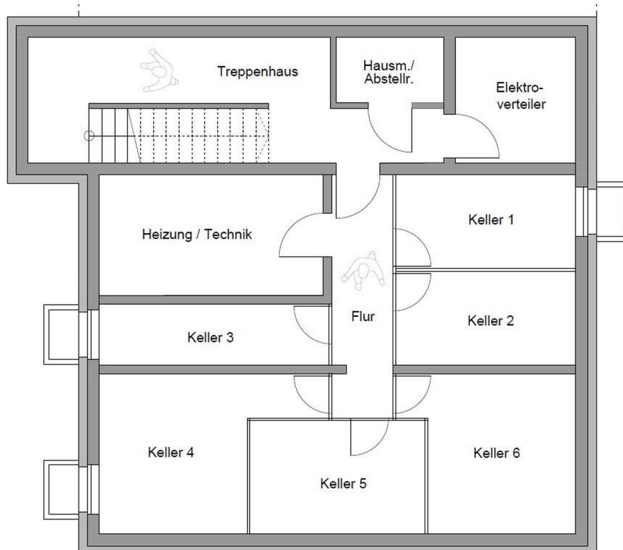
Grundriss Keller
