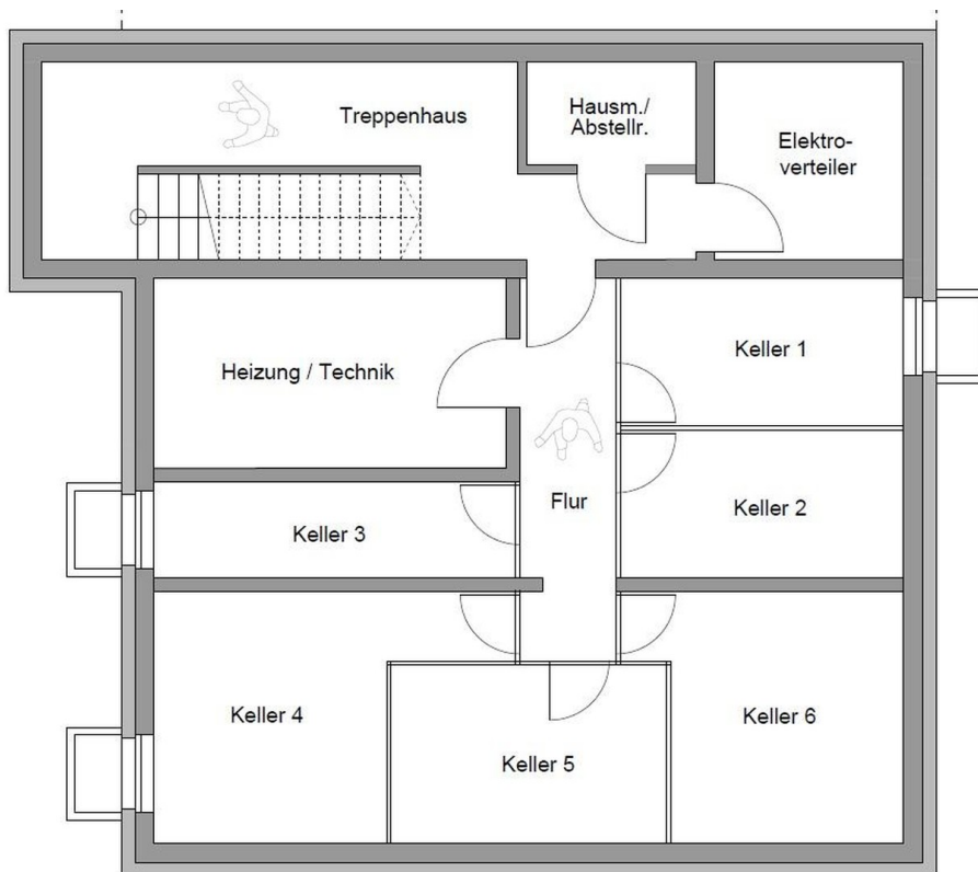
Grundriss Keller
