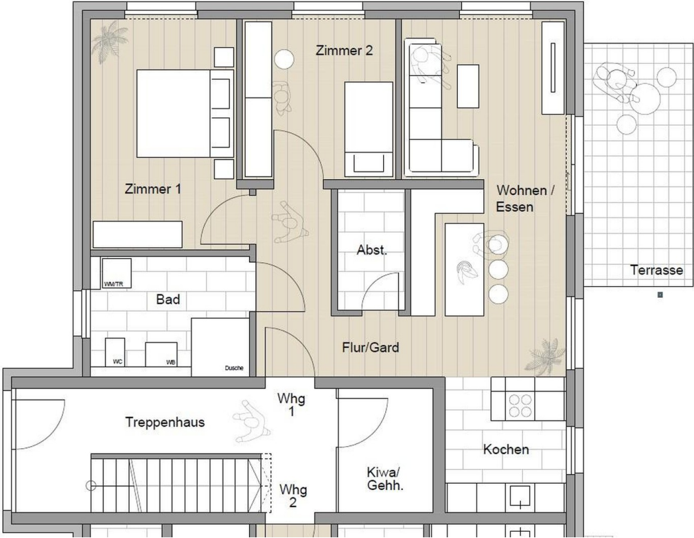
Grundriss Wohnung
