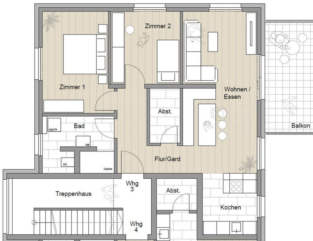
Grundriss Wohnung
