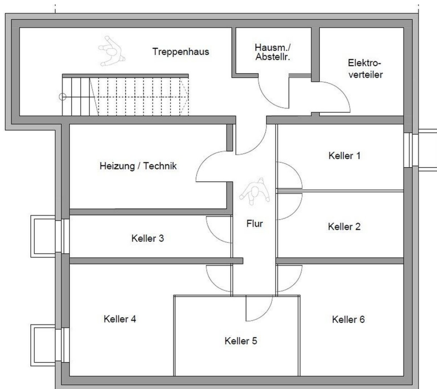
Grundriss Keller
