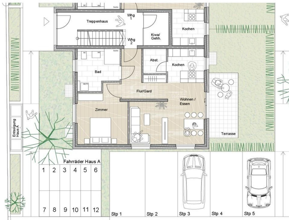
Grundriss Wohnung
