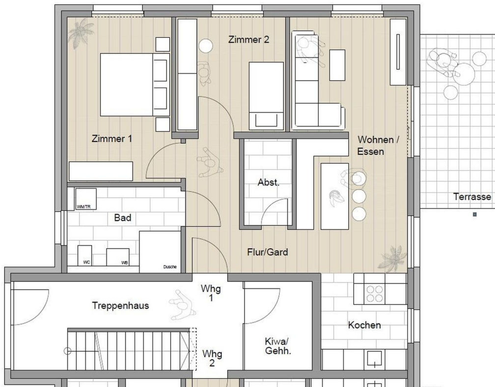
Grundriss Wohnung
