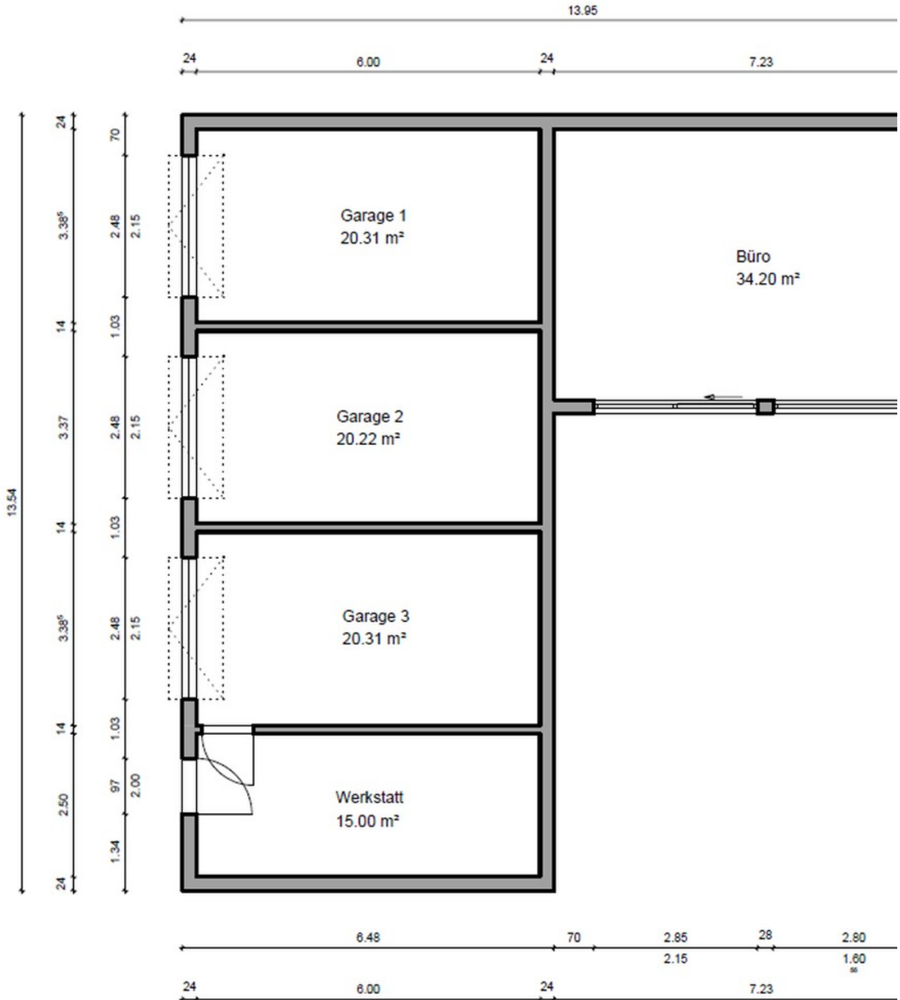
Garage & Nebengebäude
