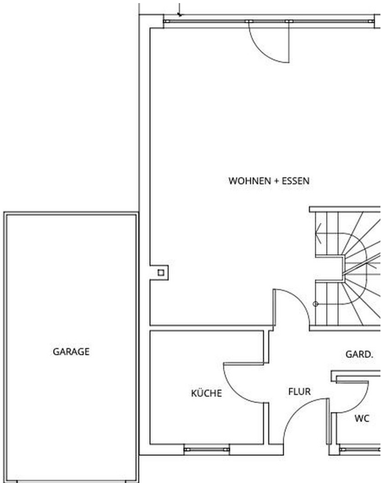
Erdgeschoss
