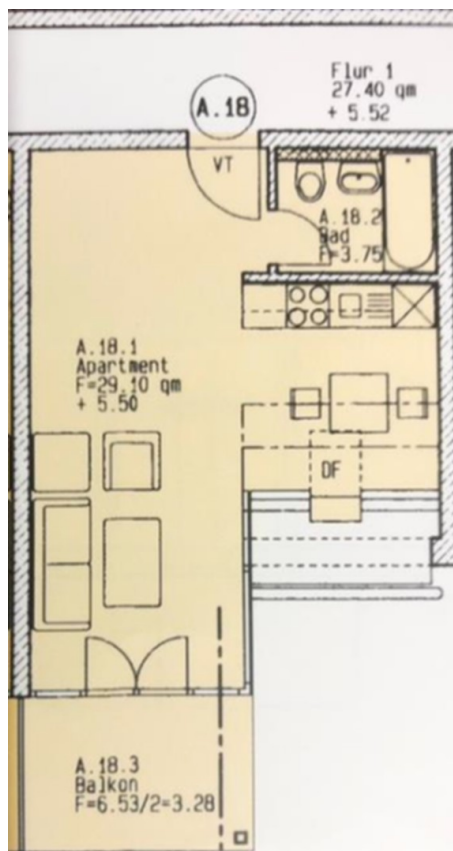
Grundriss
