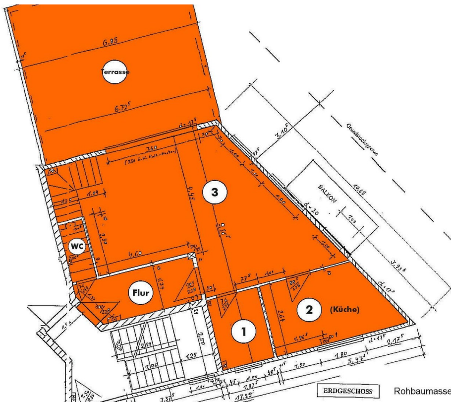
Grundriss Erdgeschoß
