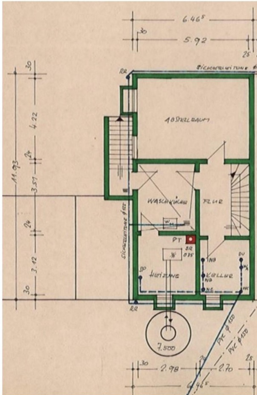
Grundriss UG (nicht maßstabstreu)
