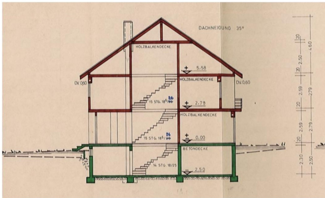
Schnitt (nicht maßstabsgetreu)
