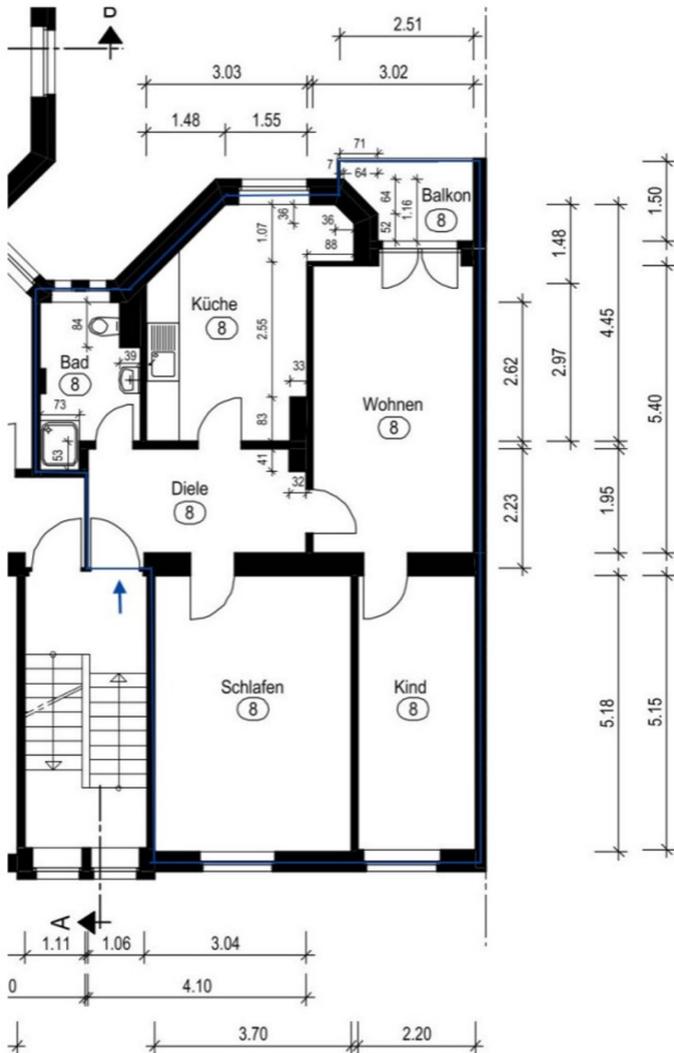
Grundriss
