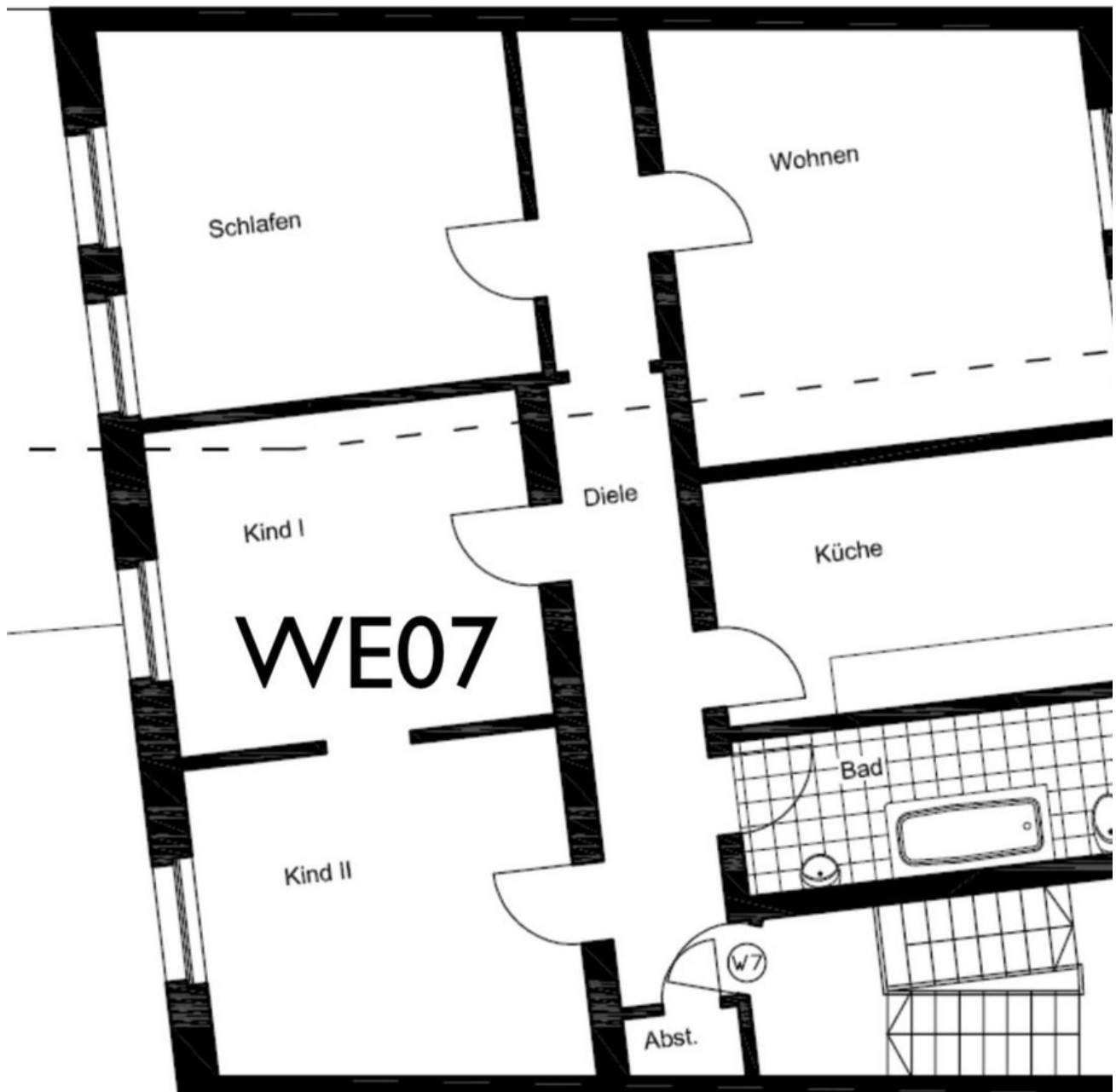
Grundriss
