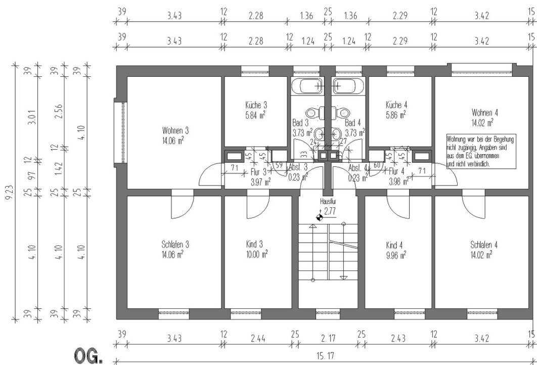
Obergeschoss - Wohnung №3
