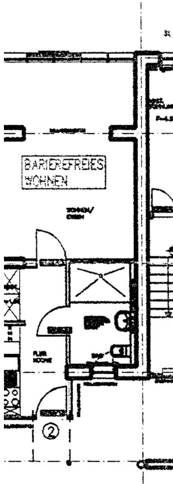
Grundriss Appartement
