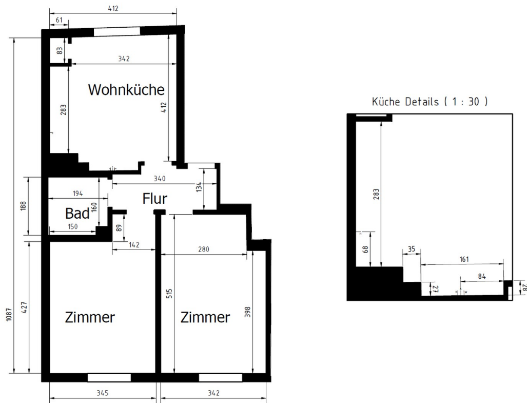
Grundriss
