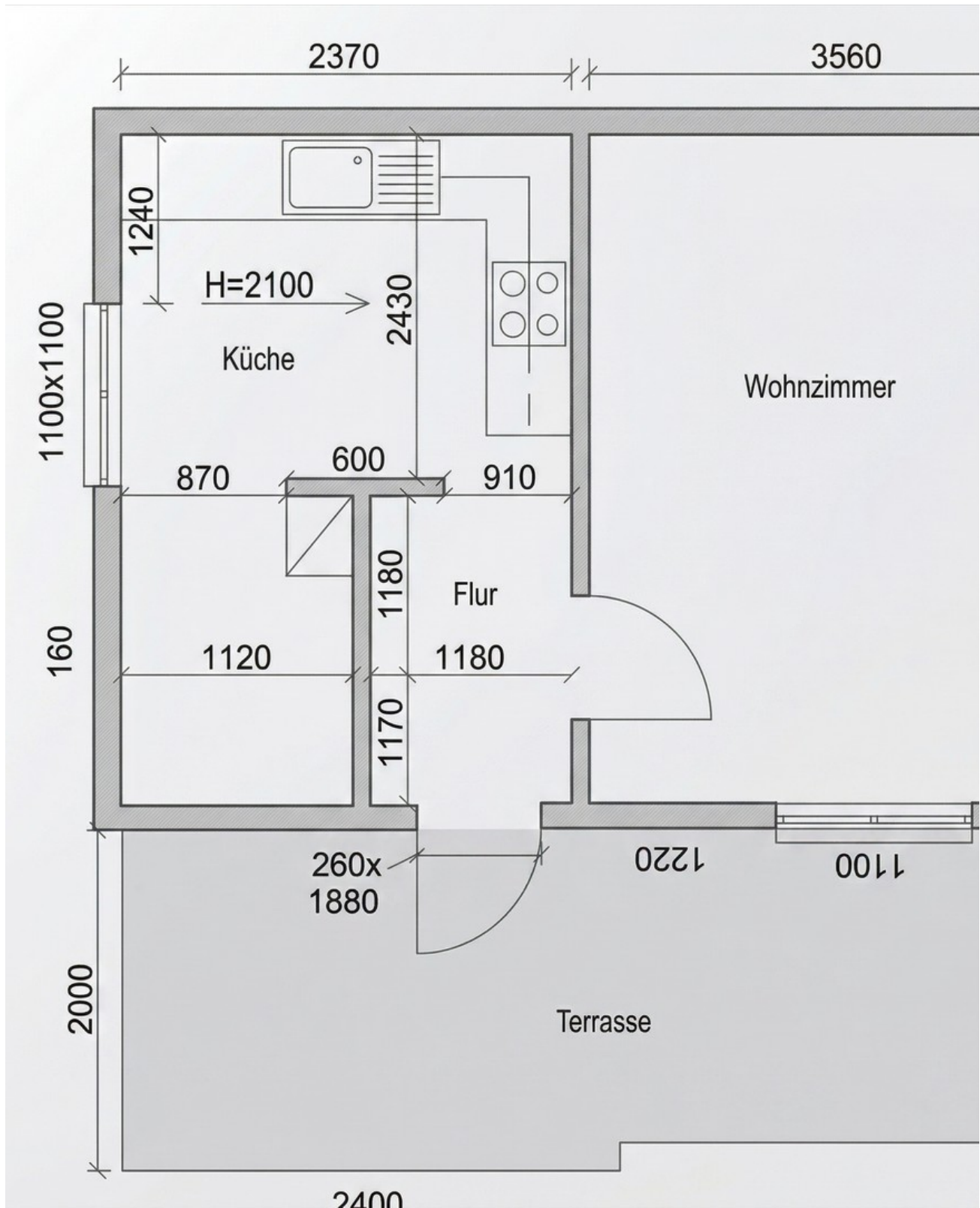
Grundriss Bklockhaus 1
