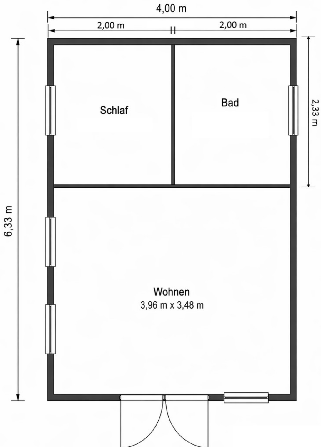
Grundriss Blockhaus 2
