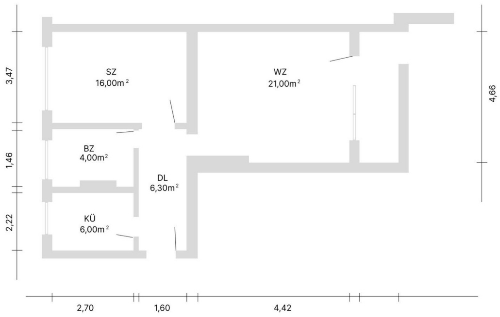
Grundriss
