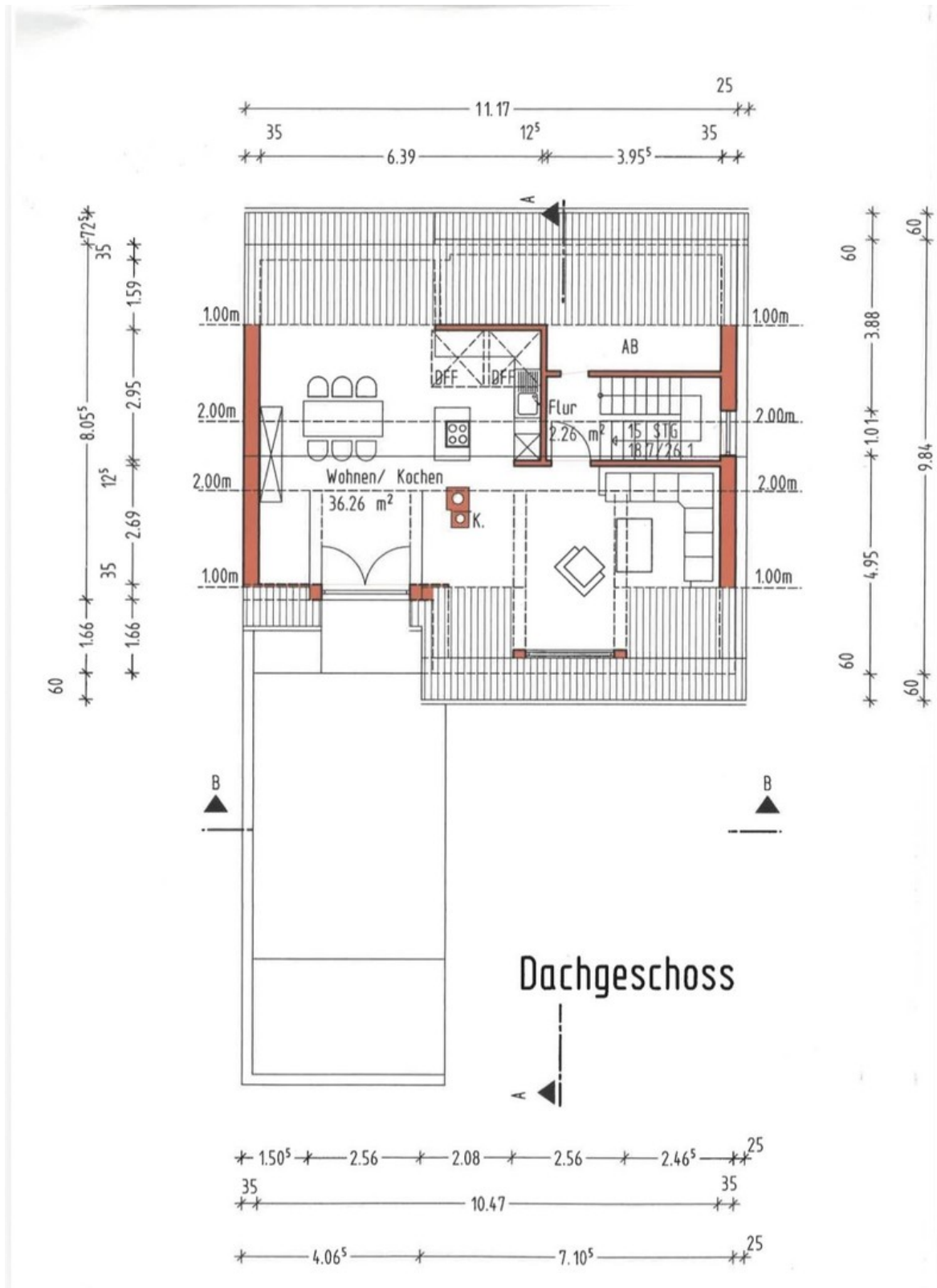
Grundriss Dachgeschoss
