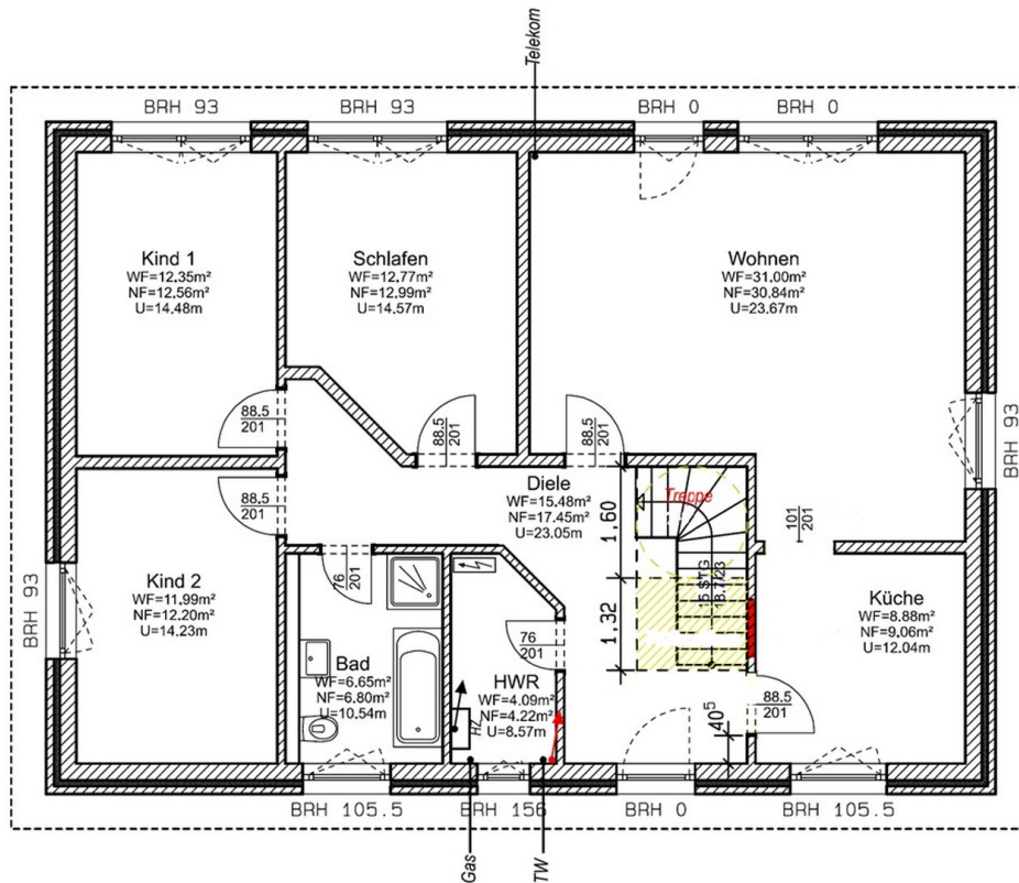
Grundriss Erdgeschoss
