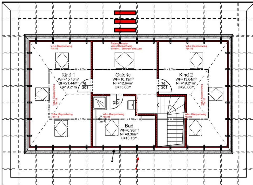
Grundriss Obergeschoss
