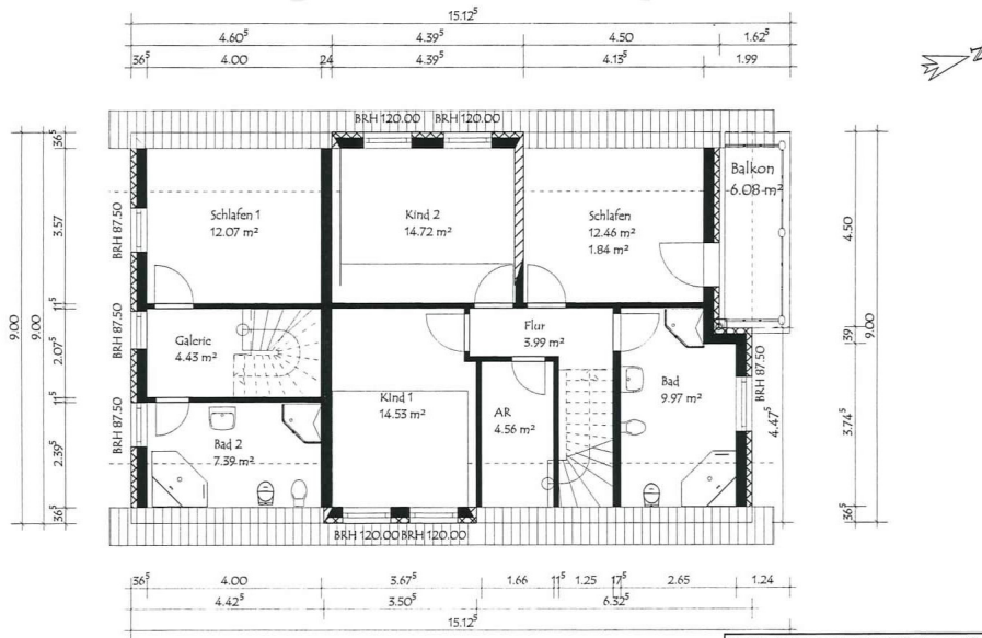
Dachgeschoss M1:100
